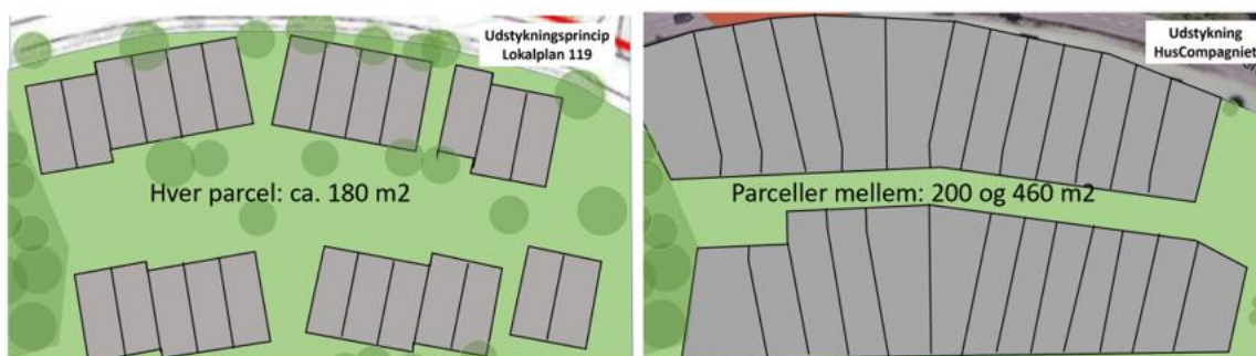
Figur 9: Udstykning i ens parceller
